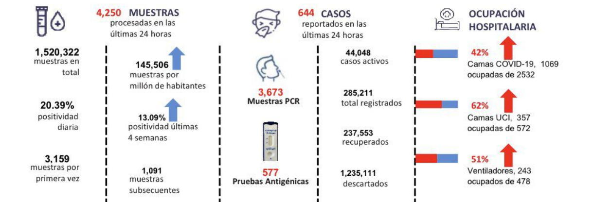
Figura 1. Tendencia de los casos v positividad de COVID-19 en República Dominicana
